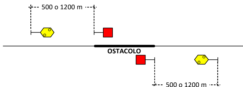
Segnalamento di fermata notificata su linea a semplice binario.
