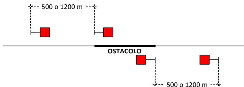
Segnalamento di fermata non notificata su linea a semplice binario.
