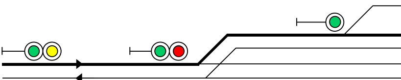
Transito per itinerario con due diramazioni successive aventi il primo deviatore disposto per il ramo deviato (30 km/h) e il secondo per il corretto tracciato.
