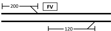
GRANDATE - BRECCIA
