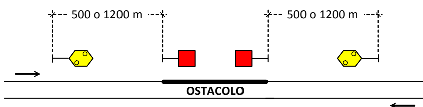
Segnalamento di fermata notificata su linea a doppio binario con ostacolo che interessa un solo binario.
